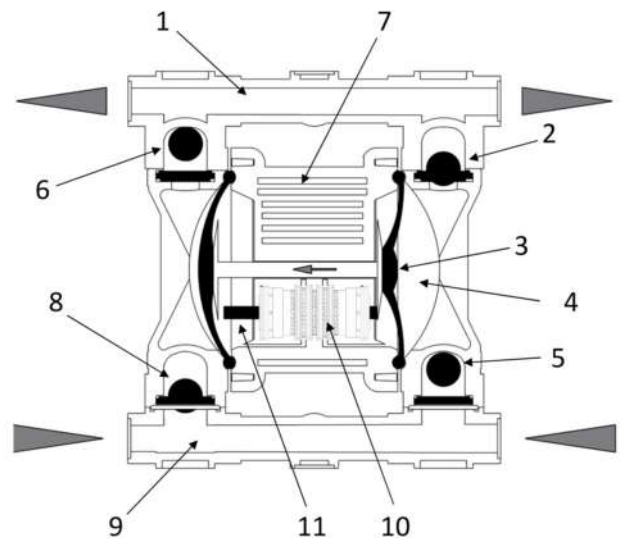
Εικ.2 Διάταξη αντλίας
