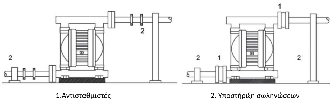
Σχήμα 3. Πρόταση εγκατάστασης Διαφραγματικής αντλίας
