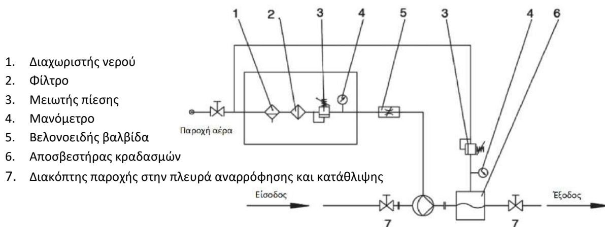
Σχήμα 3. Πρόταση εγκατάστασης Διαφραγματικής αντλίας
