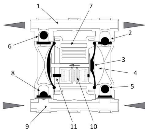
Εικ.2 Διάταξη αντλίας
