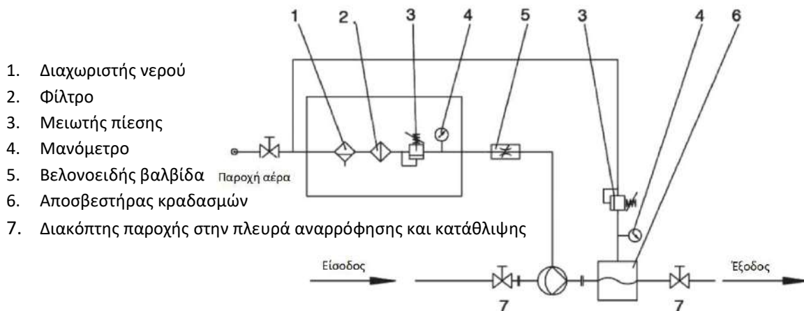
Σχήμα 3. Πρόταση εγκατάστασης Διαφραγματικής αντλίας
