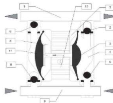
Рис. 2: Конструкция насоса
