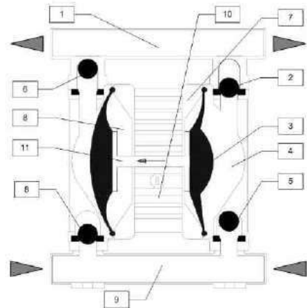
fig.2 Diseño de la bomba
